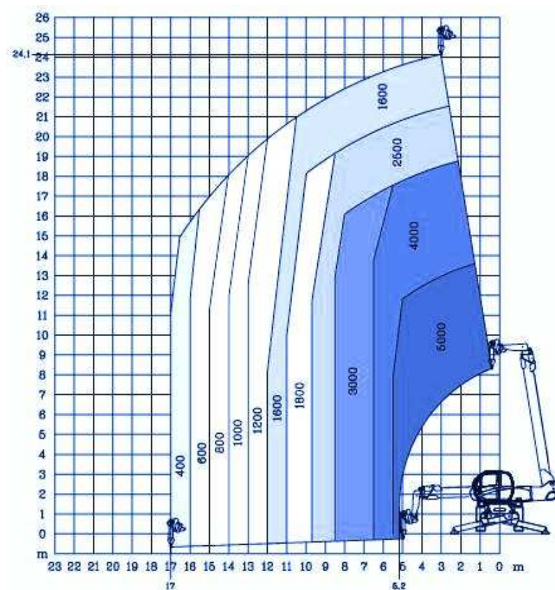
Roto 25 treuil 5Tonnes
