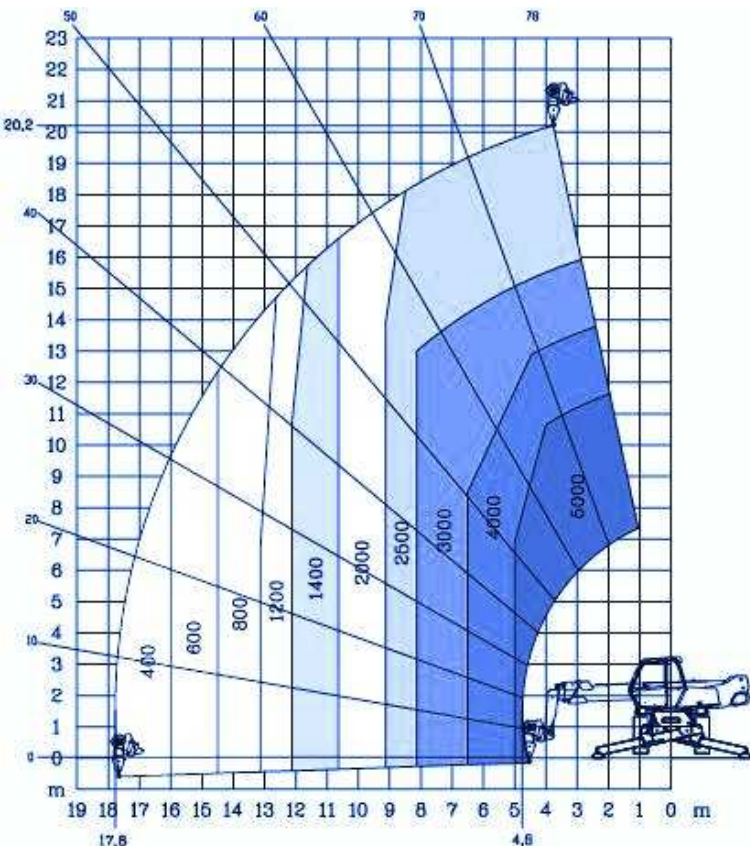
Roto 21 treuil 5Tonnes
