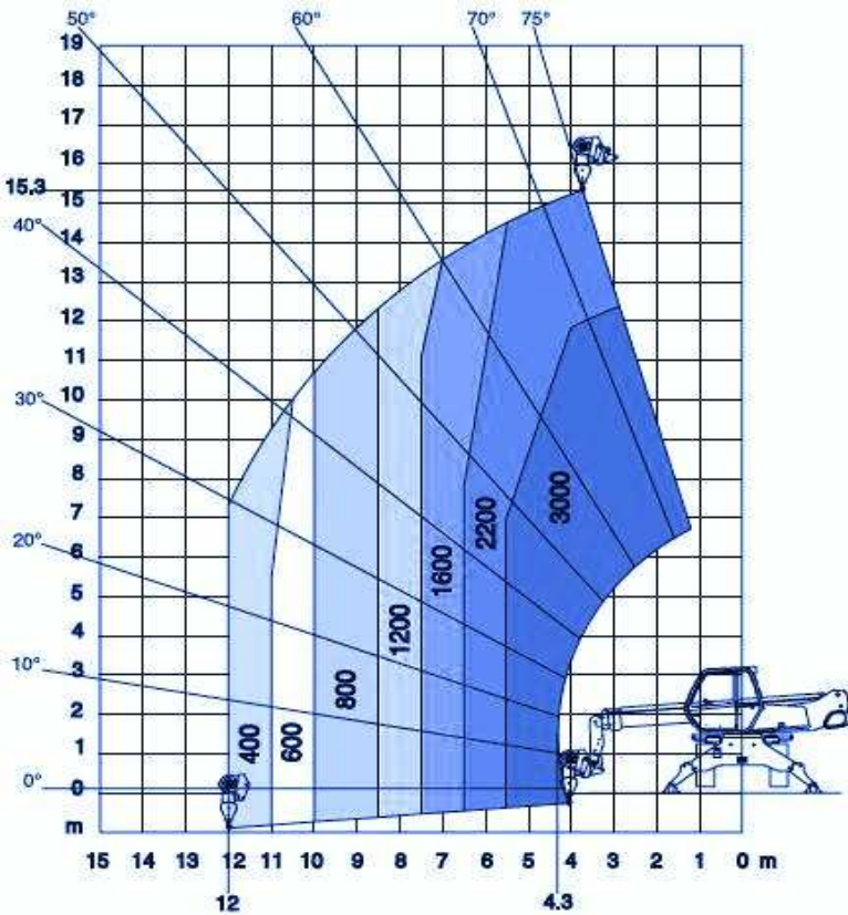
Roto 16 treuil 3Tonnes
