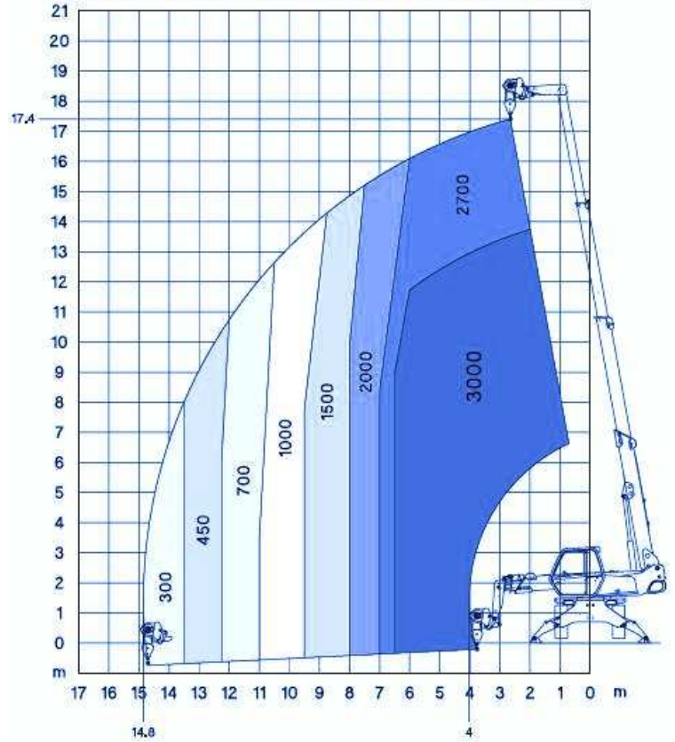
Roto 18 treuil 3Tonnes
